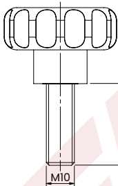
OPTIONAL HANDKNOB CODE 62200010
