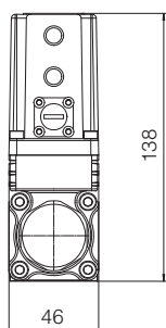
RZMO-REB-P-NP RZMO-REB-P-IL
