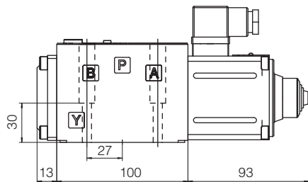
QVKZOR-A
