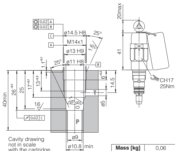
CART M-6
