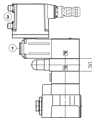
Option /P
