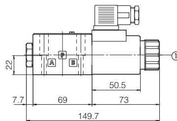
DHEP-06*/A(DC)
