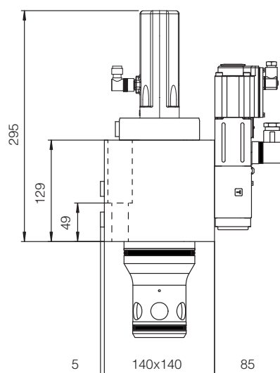
LIQZP-L-502
