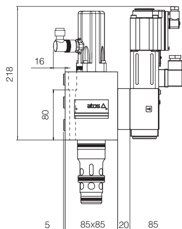
LIQZP-L-253
