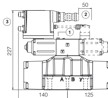
DPZO-AES-BC-2 DPZO-AES-BP-2
