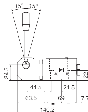
DH-01**
