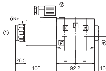
DKEP-16*/A-DC
