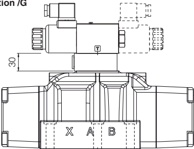
Option /G
