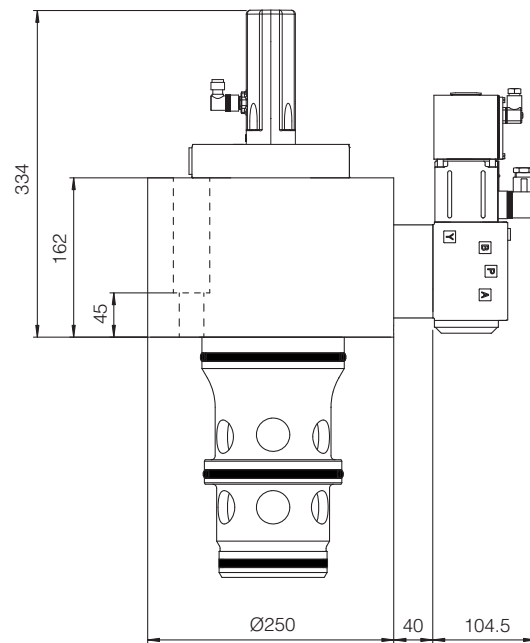
LIQZP-L-803
