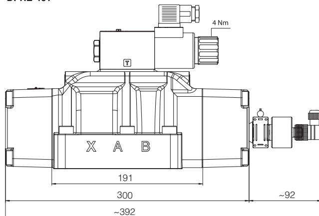
DPHE-461*
