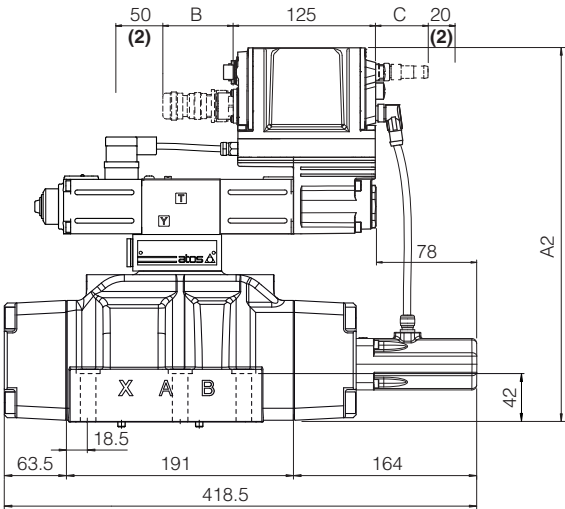
DPZO-TEB-*-47 DPZO-TES-*-47
