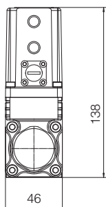
RZGO-REB-P-NP RZGO-REB-P-IL
