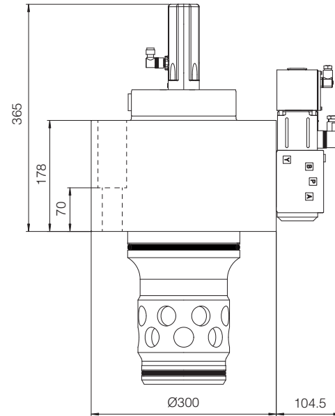
LIQZP-L-1002
