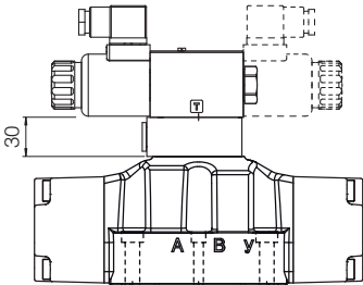
Option /G
