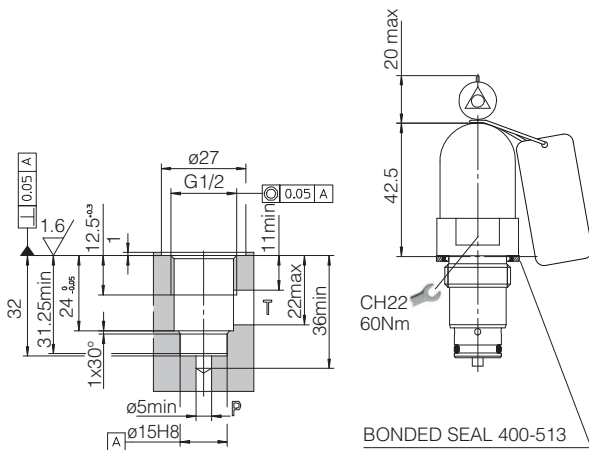
CART M-3
