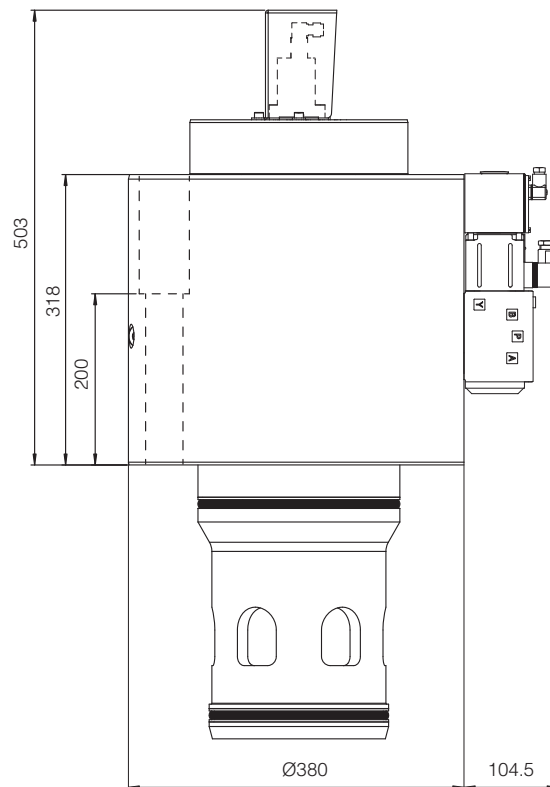
LIQZP-L-1252
