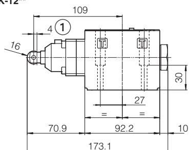
DK-12**
