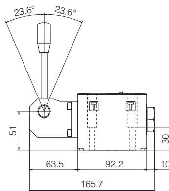
DK-11**
