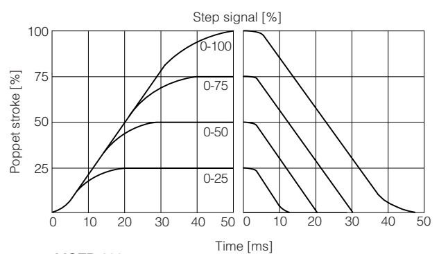
LIQZP-100
