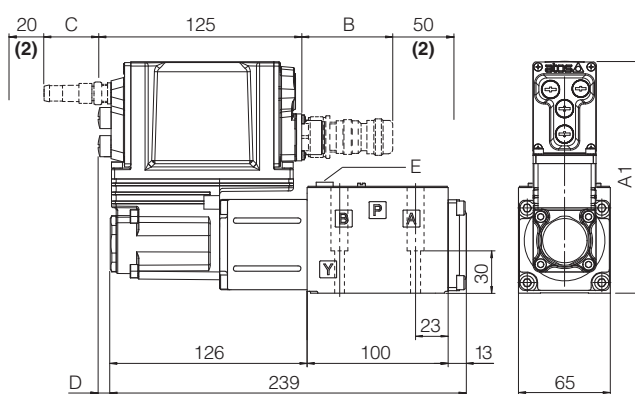
DKZOR-TEB-*15 DKZOR-TES-*15
