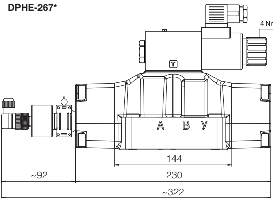
DPHE-263* DPHE-267*
