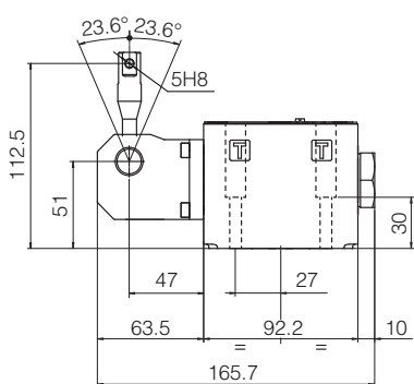
DK-12**
